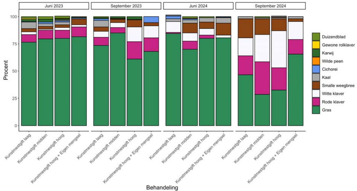
Figuur 15 Resultaat kruidentellingen deelnemer D. In 2024 (een relatief nat jaar) valt op dat de stroken aan de zijkant van het perceel minder klavers bevatten dan de middelste stroken.
