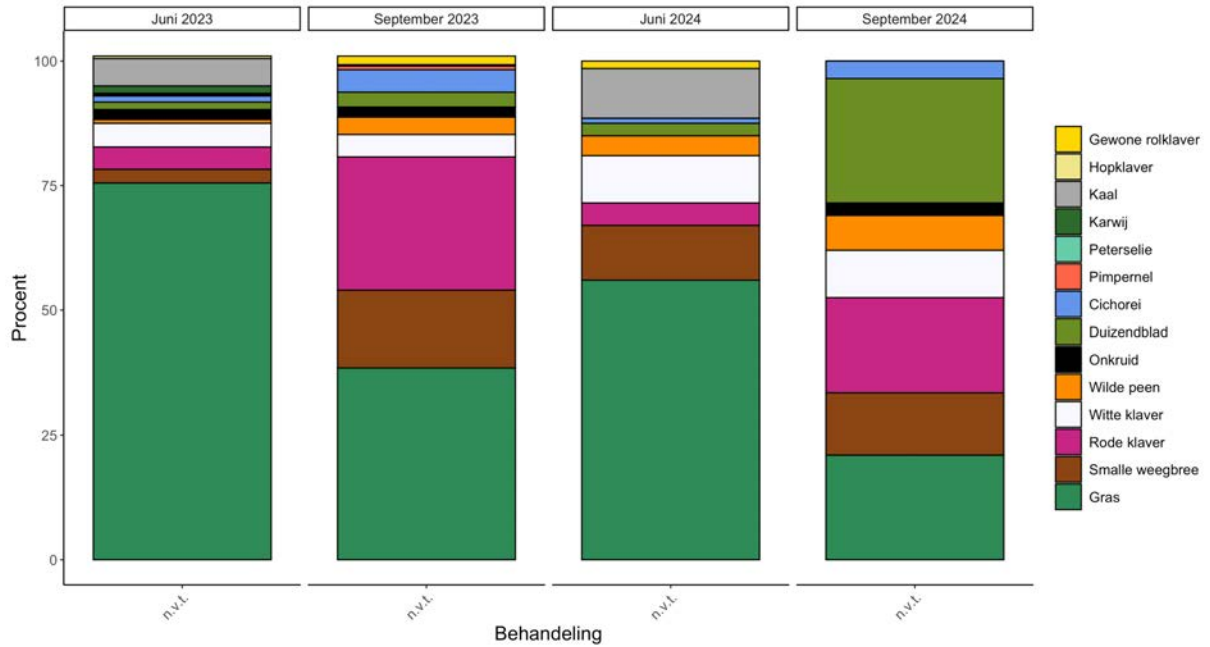
Figuur 20. Resultaat kruidentellingen deelnemer G. De toenemende diversiteit is opvallend op dit perceel.
