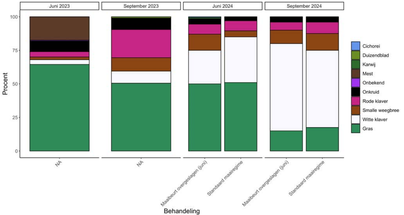
Figuur 36. Resultaat kruidentellingen bij deelnemer B. Naast grassen groeien voornamelijk klavers en kleine weegbree in dit perceel, het aandeel witte klaver nam toe over tijd. In 2024 was er geen verschil in soortensamenstelling, maar wel een verschil in het aandeel van de verschillende soorten in de vegetatie.
